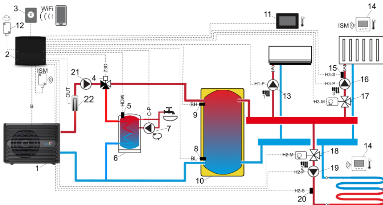
Schemat z buforem ciepła i zasobnikiem CWU 3 (funkcja chłodzenia): 1 – pompa ciepła, 2 – regulator, 3 – moduł internetowy, 4 – zawór 3-drogowy, 5 – czujnik temp. zasobnika CWU, 6 – zasobnik CWU, 7 – pompa cyrkulacji, 8 – dolny czujnik temp. bufora, 9 – górny czujnik temp. bufora, 10 – bufor ciepła, 11 – panel sterujący z funkcją termostatu pokojowego, 12 – czujnik temp. zewnętrznej (pogodowy), 13 - pompa mieszacza 1, 14 – bezprzewodowy termostat pokojowy, 15 – czujnik temp. mieszacza 3, 16 – pomp mieszacza 3, 17 – siłownik mieszacza 3, 18 – siłownik mieszacza 2, 19 – pompa mieszacza 2, 20 – czujnik temp. mieszacza 2, 21 – pompa CWU, 22 – grzałka przepływowa.
